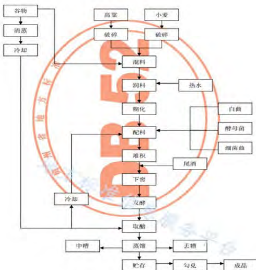
图2 麸曲酱香型白酒生产工艺流程图
